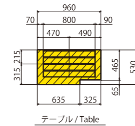
テーブル / Table
