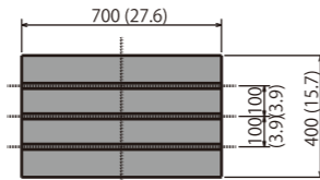
テーブル寸法図 / Table
