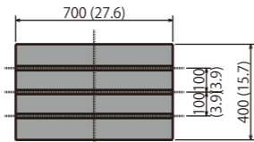
テーブル寸法図 / Table
