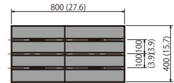
テーブル寸法図 / Table
