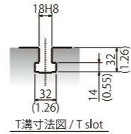
T溝寸法図 / T slot
