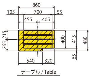
テーブル / Table
