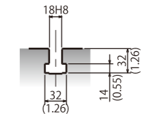
T溝寸法図 / T slot
