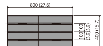
テーブル寸法図 / Table
