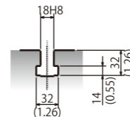
T溝寸法図 / T slot
